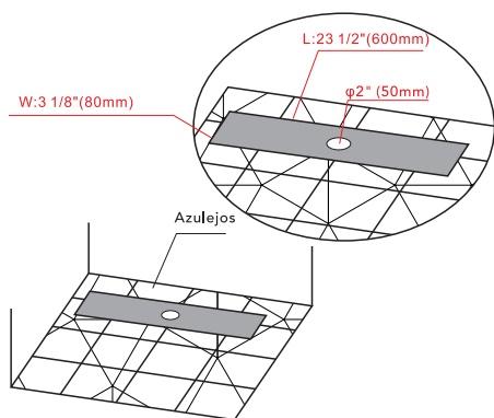
Piso del baño inclinado Vista desde arriba
