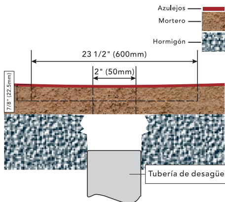
Diagrama de sección transversal del piso
